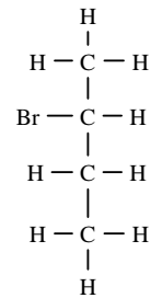
R-2-Brom-Butan (L-Form)
