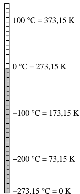
relative und absolute Temperaturskala am Gasthermometer
